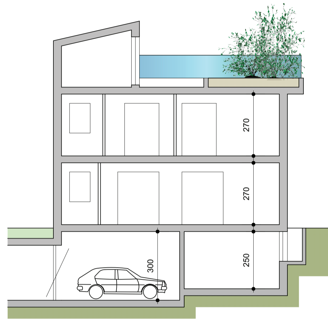
SEZIONE
